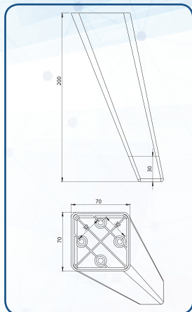
MANGO (70x70X200) mm 111353101121461 Ağa -Krom
