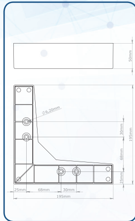
GÖKNAR (195x195x50) mm 111105812121462 Ağaç
