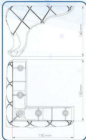
OKALIPTUS (170x170x140) mm Taşlı 111128312151162 Beyaz
