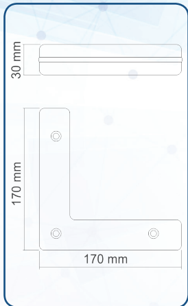
PELESENK (170x170x30) mm 11115512121362 Ağaç
